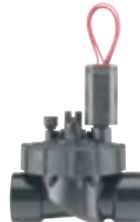
PGV-101JT - G Średnica wejścia: 1" Wysokość: 14 cm Długość: 11 cm Szerokość: 8 cm
