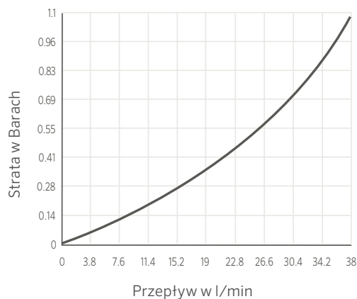
STRATY WSKUTEK TARCIA NA POŁĄCZENIU RUCHOMYM
