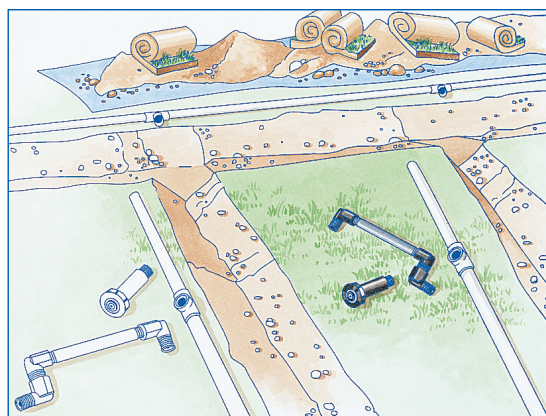
Ułóż rury i zraszacze w pobliżu wykopów zgodnie ze sposobem ich instalacji.
